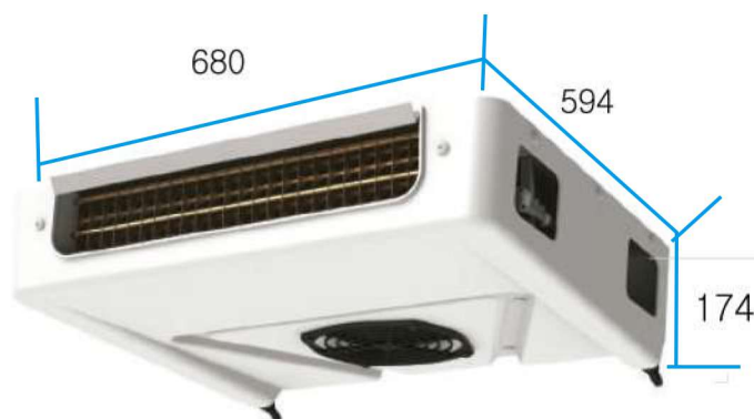
Evaporador Dimensiones 680×594×174(L×W×H/mm)
